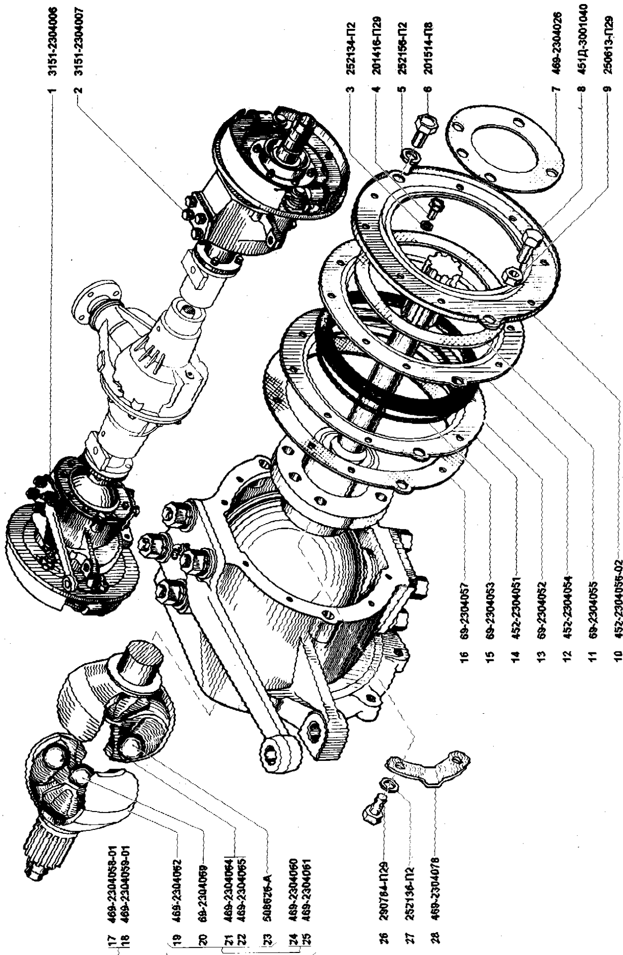
Рис. 68. Кынакч нарворотныя (2304)/1 Fig. 68. Steering knuckles (2304)/1
